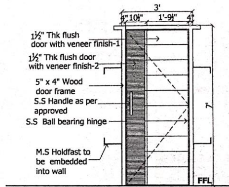
ELEVATION - D1 (3'-0" x 7'-0")
